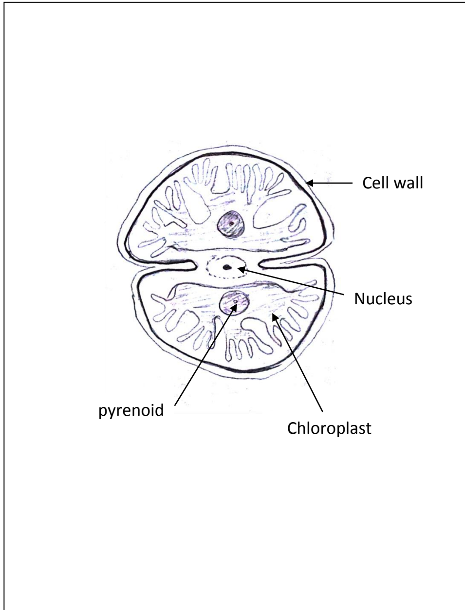
G : Cosmarium
