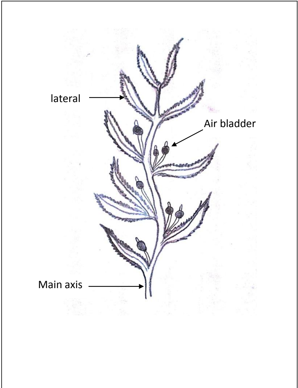
G : Sargassum
