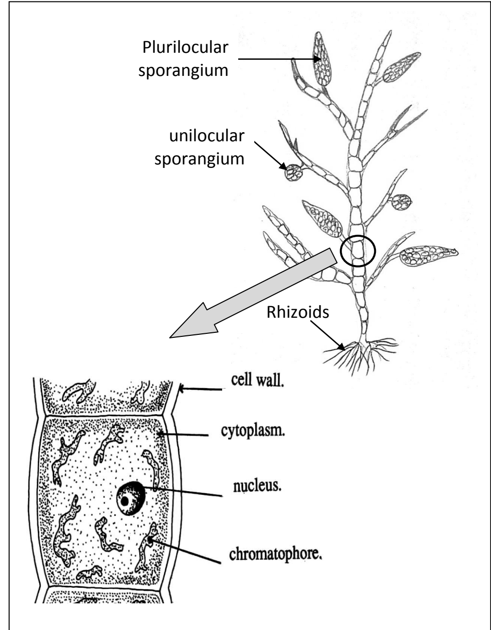
G : Ectocarpus
