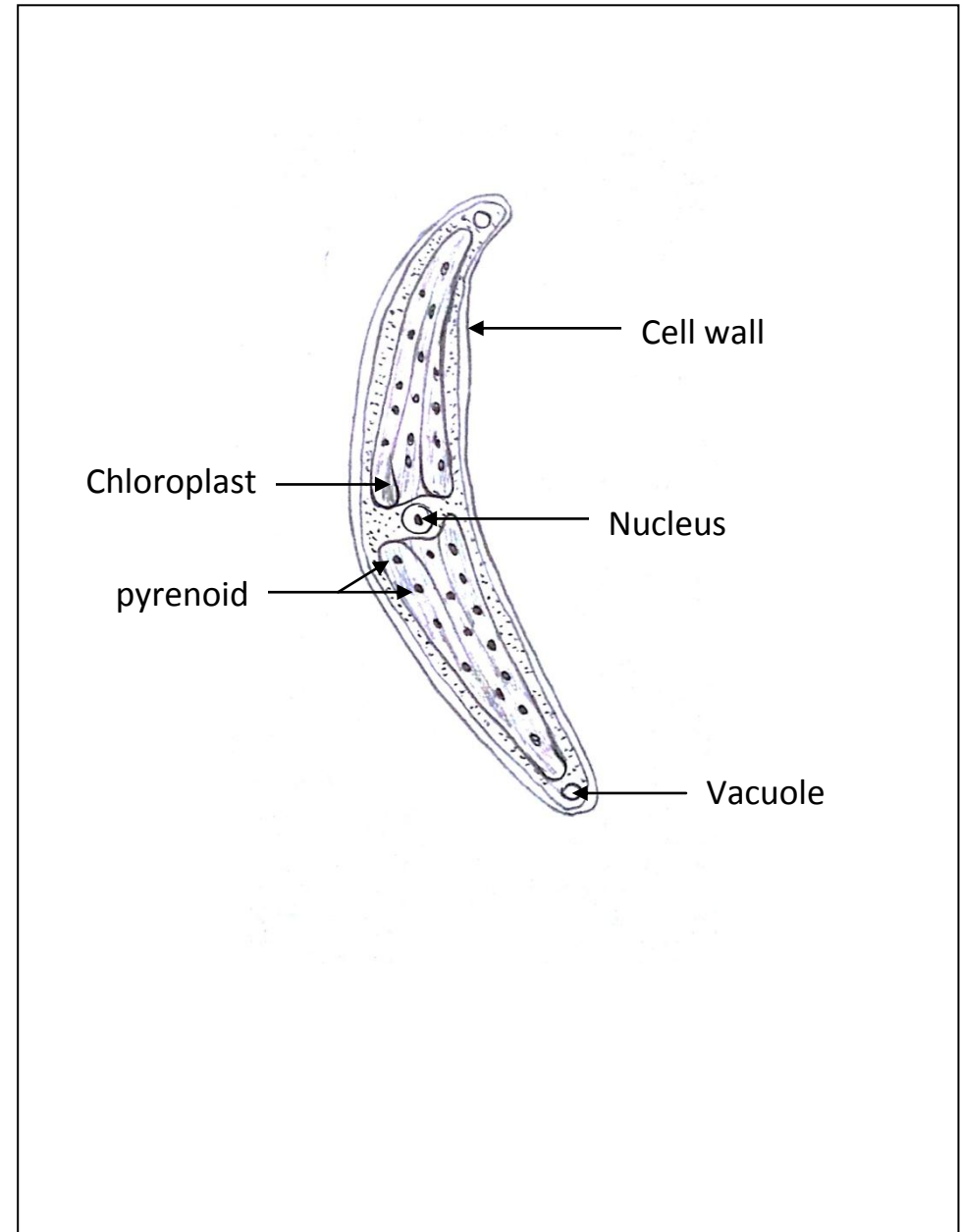
G : Closterium
