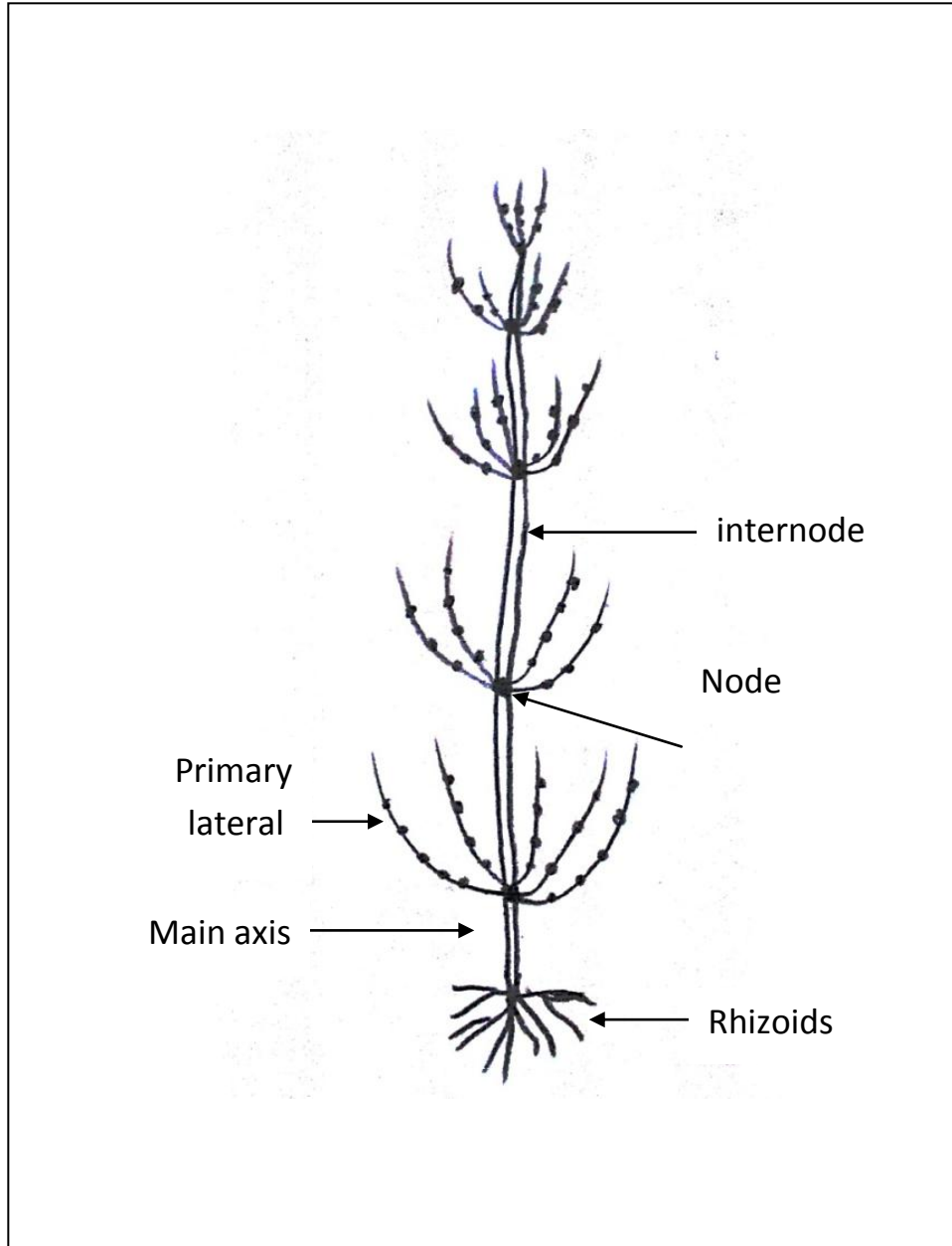
G : Chara
