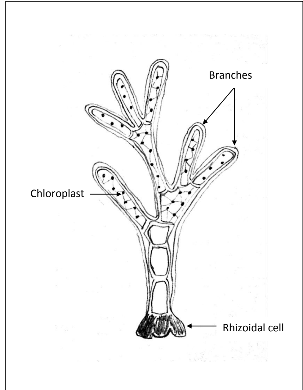
G : Cladophora
