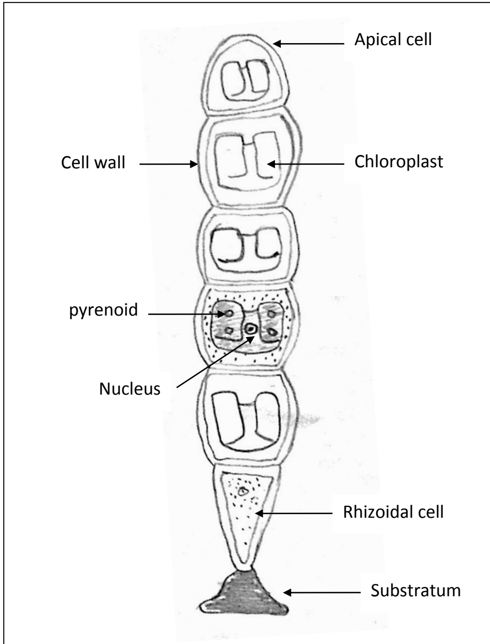
G : Ulothrix
