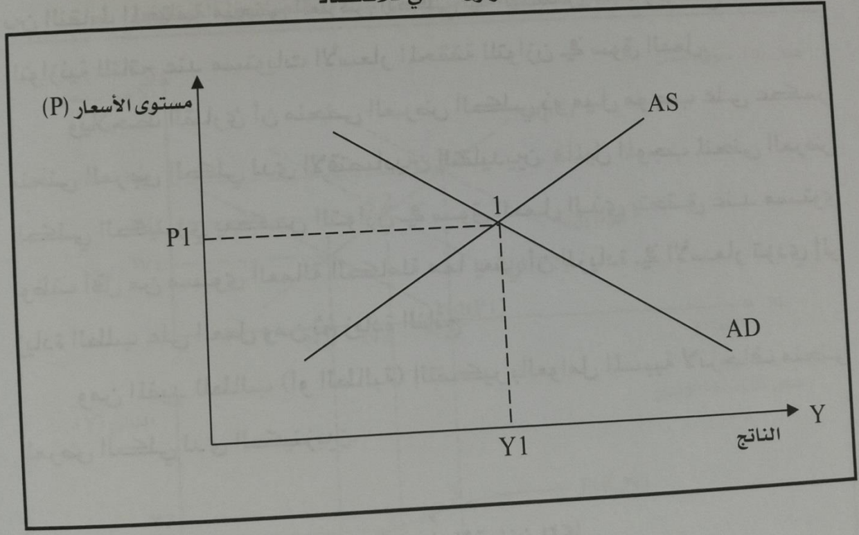
شكل رقم (6) التوازن الكلي للاقتصاد
