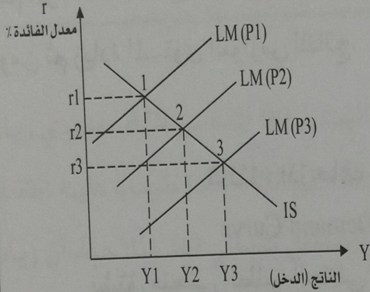
نموذج IS - LM
