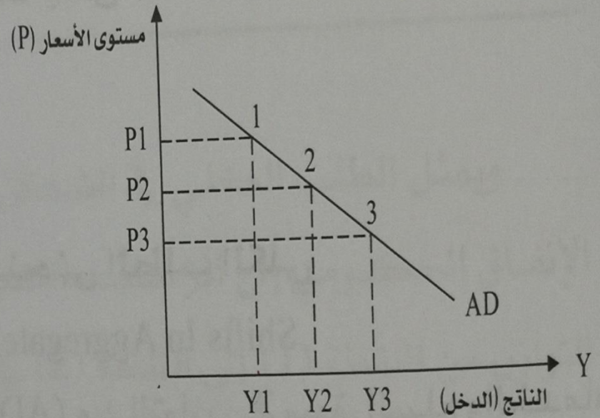
منحني الطلب الكلي
