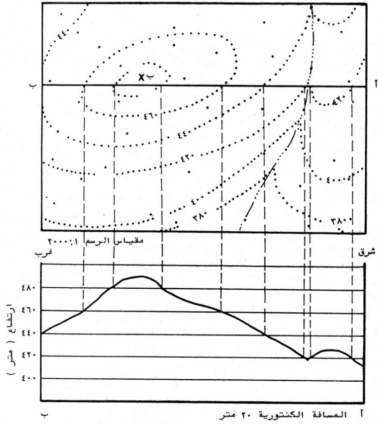
شكل ( ٢ - ٣ ) طريقة توصيل خطوط المناسيب والمسافة الكنتورية
