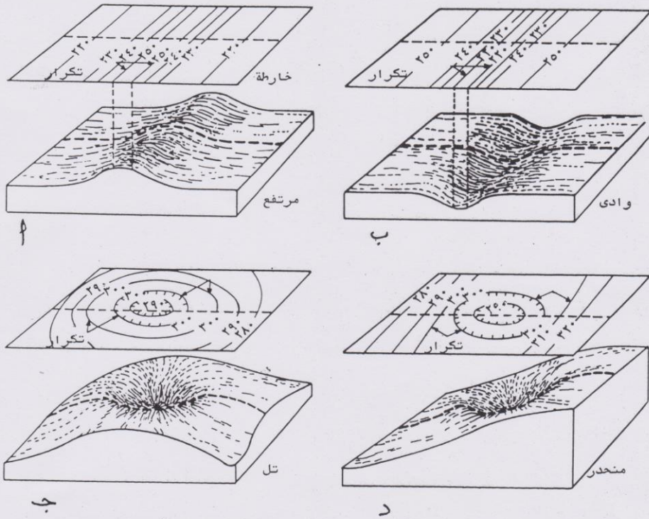
شكل (٢ - ٤) كيفية ترقيم خطوط الكنتور
