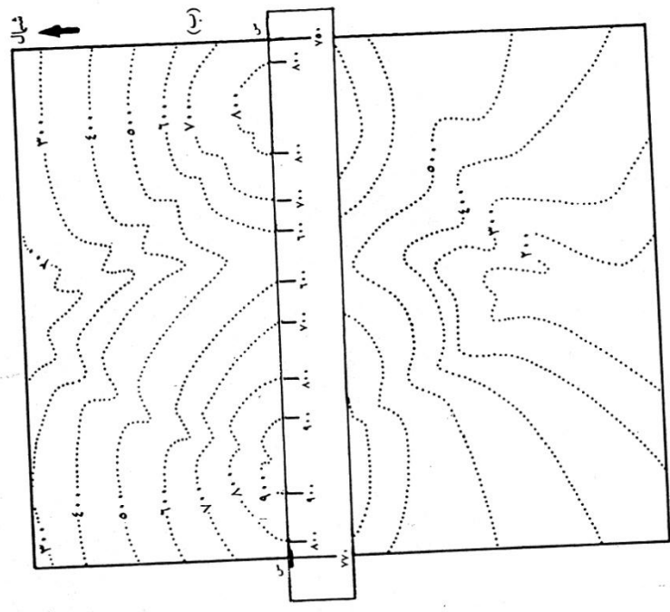
مقياس الرسم : ١ : ١٠,٠٠٠ شكل ٩ . (ب) وضع شريط من الورق بين النقطتين س من لتحديد التقاطعات بين شريط الورق وخطوط المناسيب.
