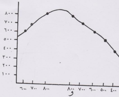
شكل ( ٢ - ١٠ ) يوضح طريقة رسم المقطع الطبوغرافى
