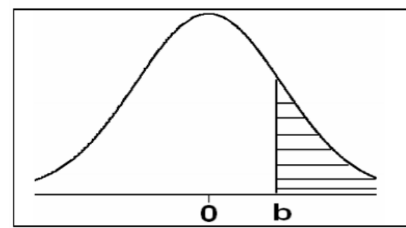
P(Z \geq b) = 1 - P(Z \leq b)
