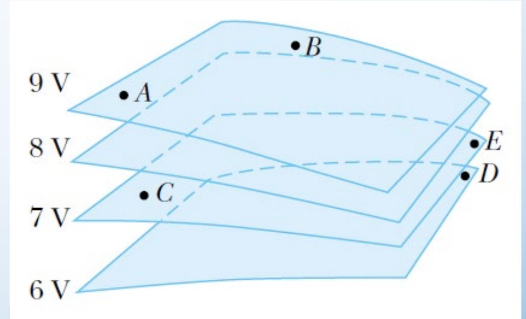
Four equipotential surfaces.
