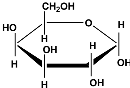
D-Galactose
