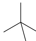
Neopentane b.p 10^\circ\text{C} m.p -17^\circ\text{C}
