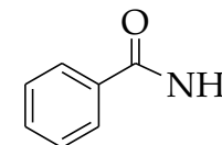
Benzamide
