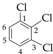
1,2,3-Trichlorobenzene
