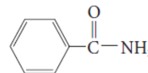
benzamide (benzenecarboxamide)
