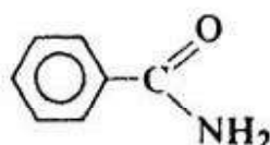
Benzamide
