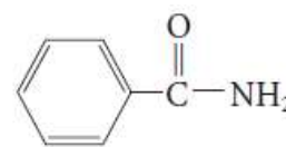
benzamide (benzenecarboxamide)
