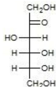
D-Fructose
