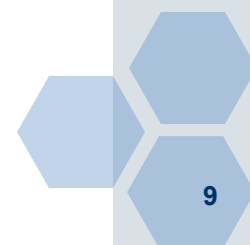
D-galactose
