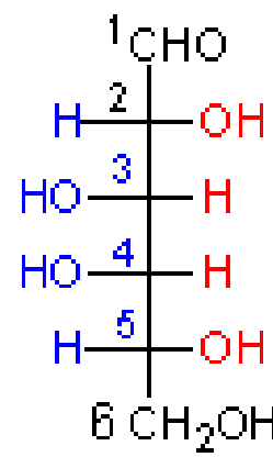
D-galactose
