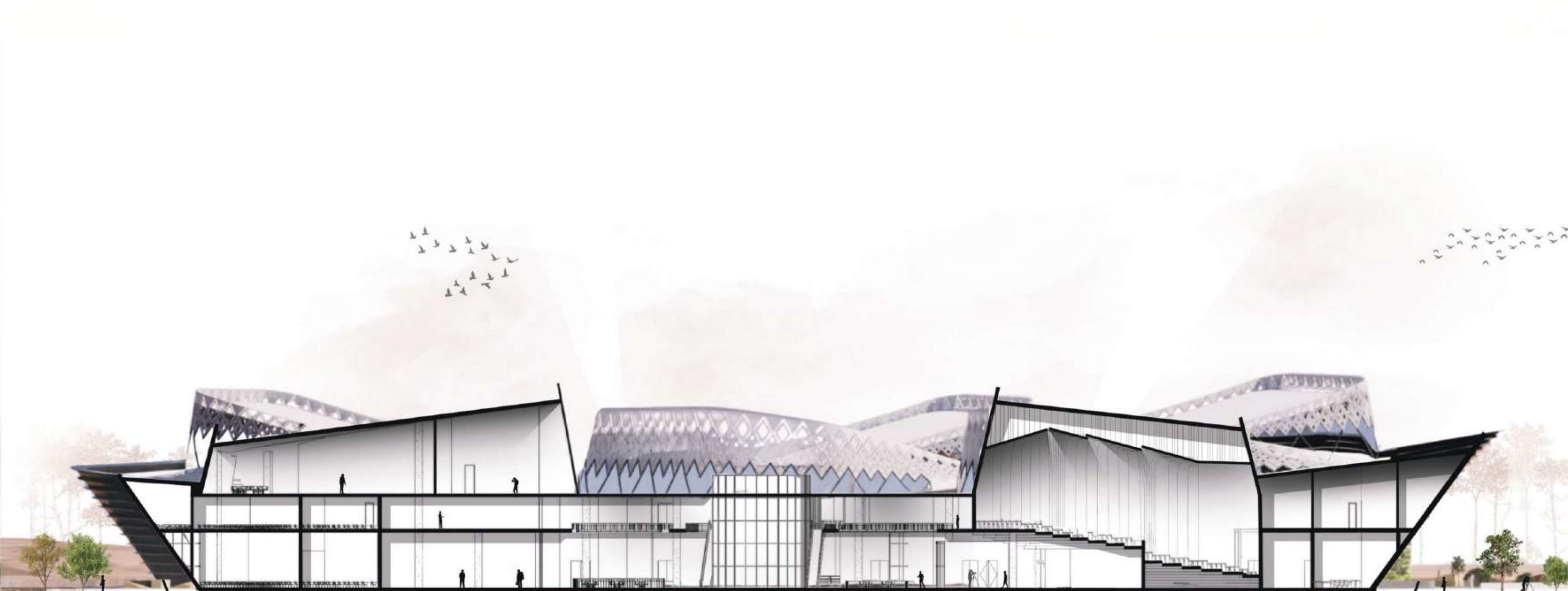
القطاع أ-أ s : 1/200
