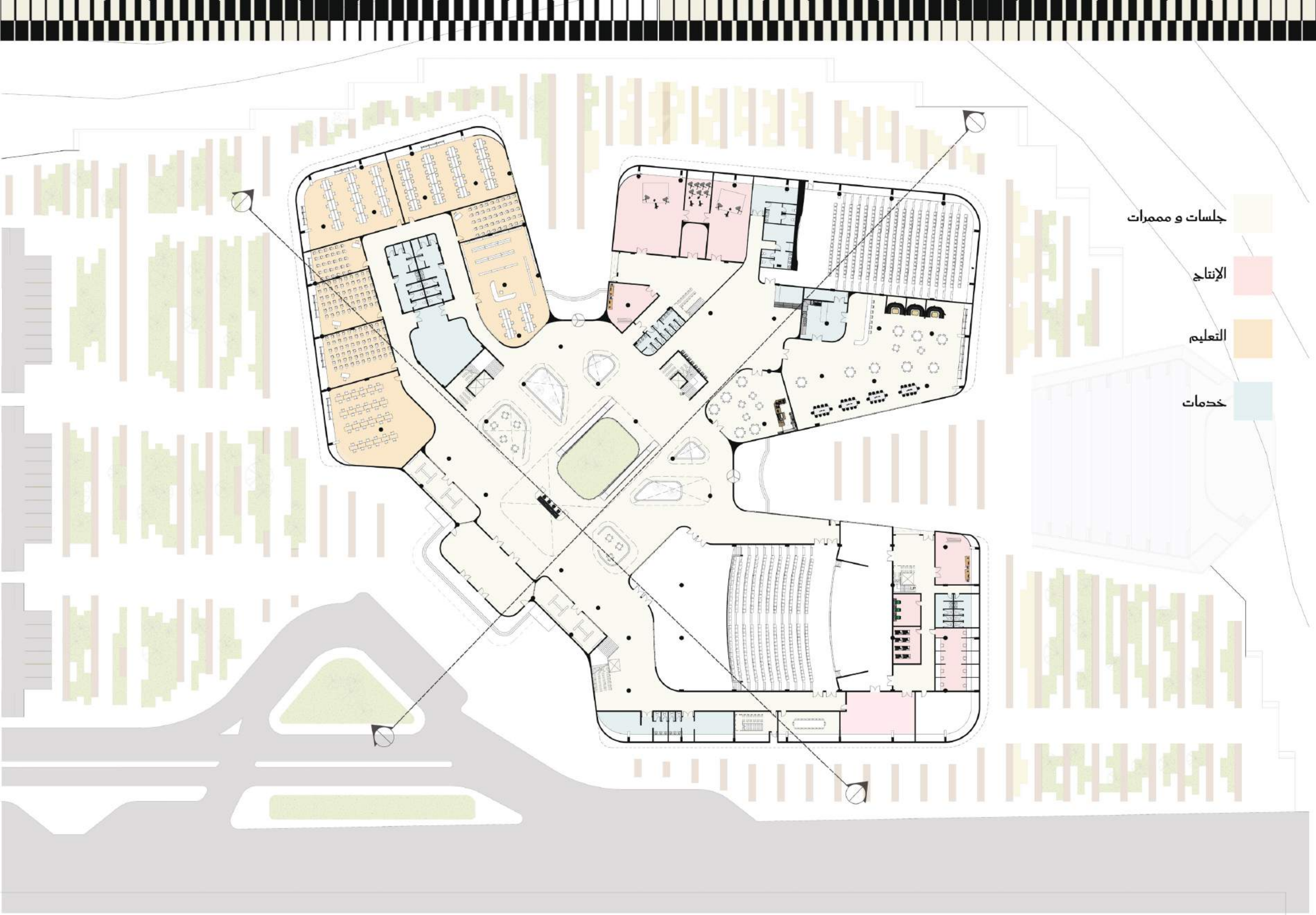
مسقط الطابق الأرضي
