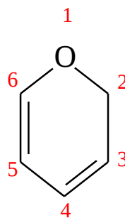
2H-Pyran
