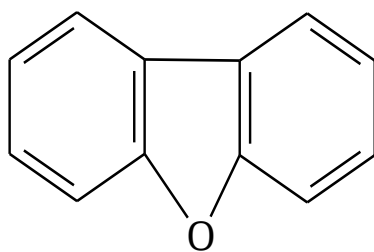
Dibenzo[b,d]oxole
