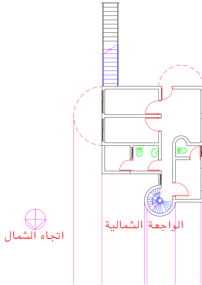
اسقاط صحيح لخطوط الواجهة الشمالية
