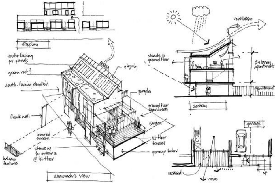
شكل (١١): اسكتشات يدوية لمبنى سكني، مع توضيح للفكرة الأساسية في التصميم القائمة على توجيه المبنى، وتوظيف حركة الرياح. المصدر: موقع دلا للعمارة التنفيذية ١٧ .
