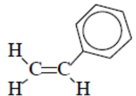
Styrene
