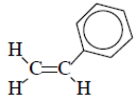
Styrene
