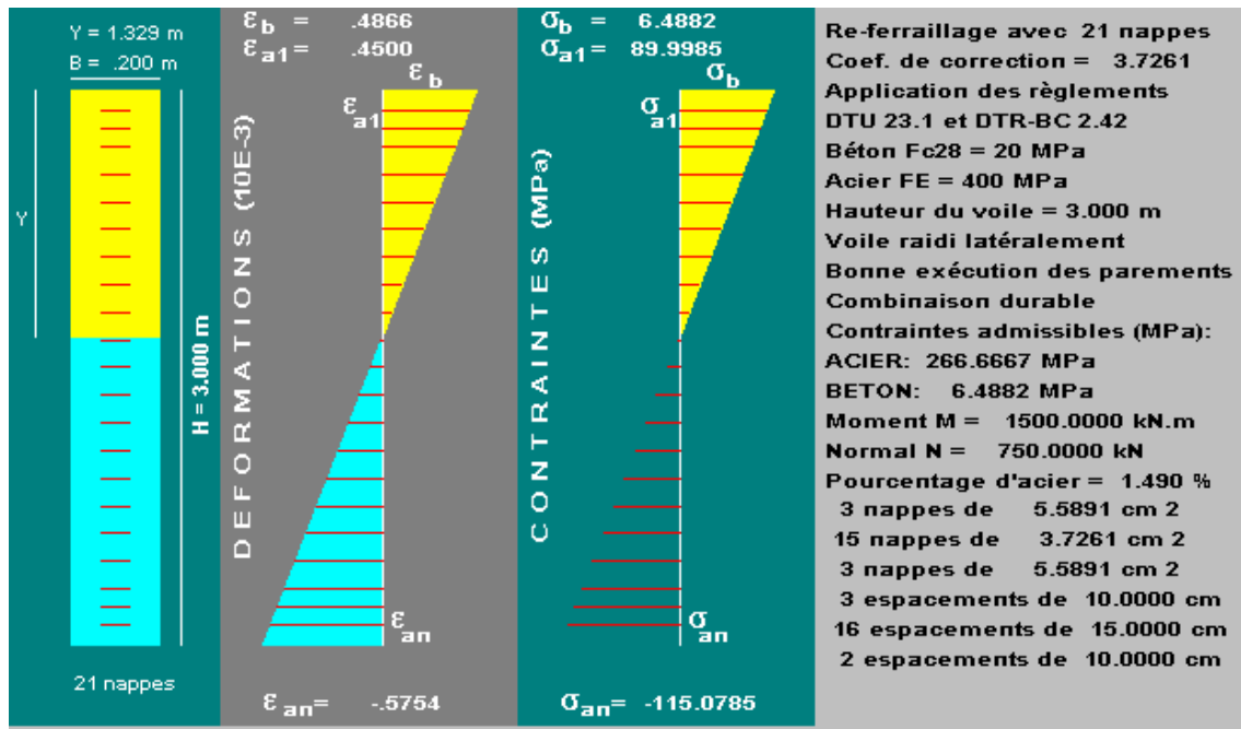
Ferraillage des voiles avec des nappes et espacements quelconques
