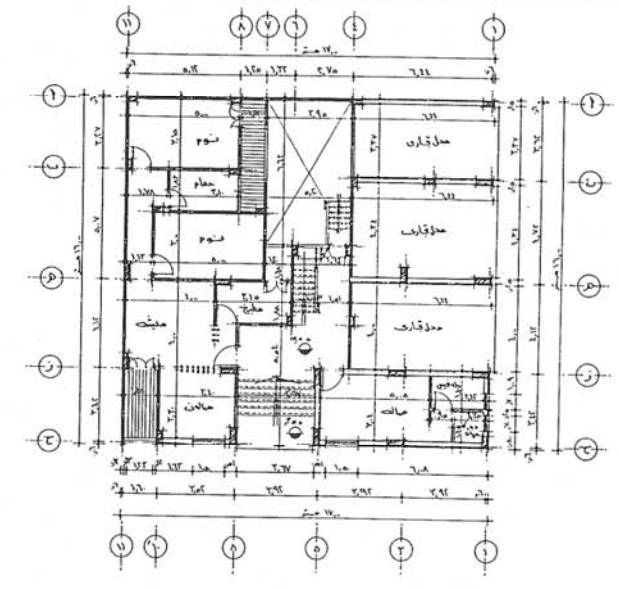
مسقط أفقى للدور الأرضى
