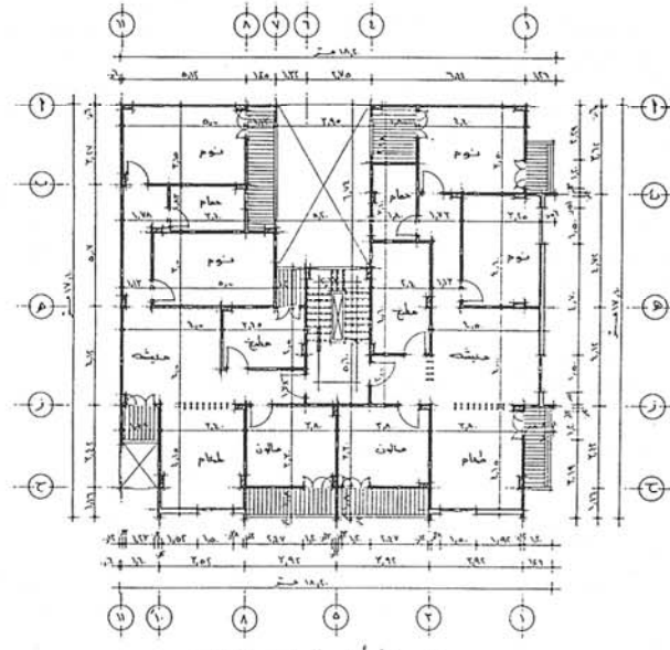
مسقط أفقى للدور المتكرر
