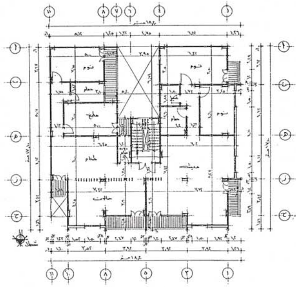
مسقط أفقى للدور الأول العلوى
