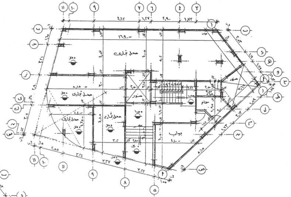
مسقط أفقى للدور الأرضى
