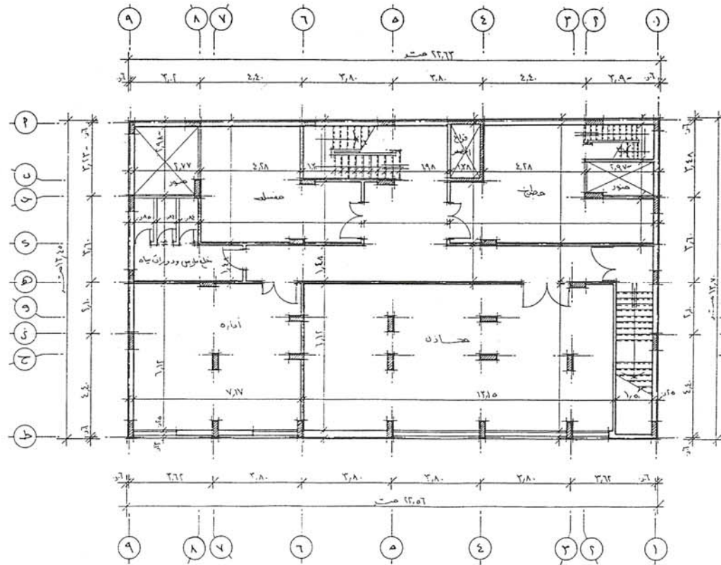
مسقط أفقى للبدروم
