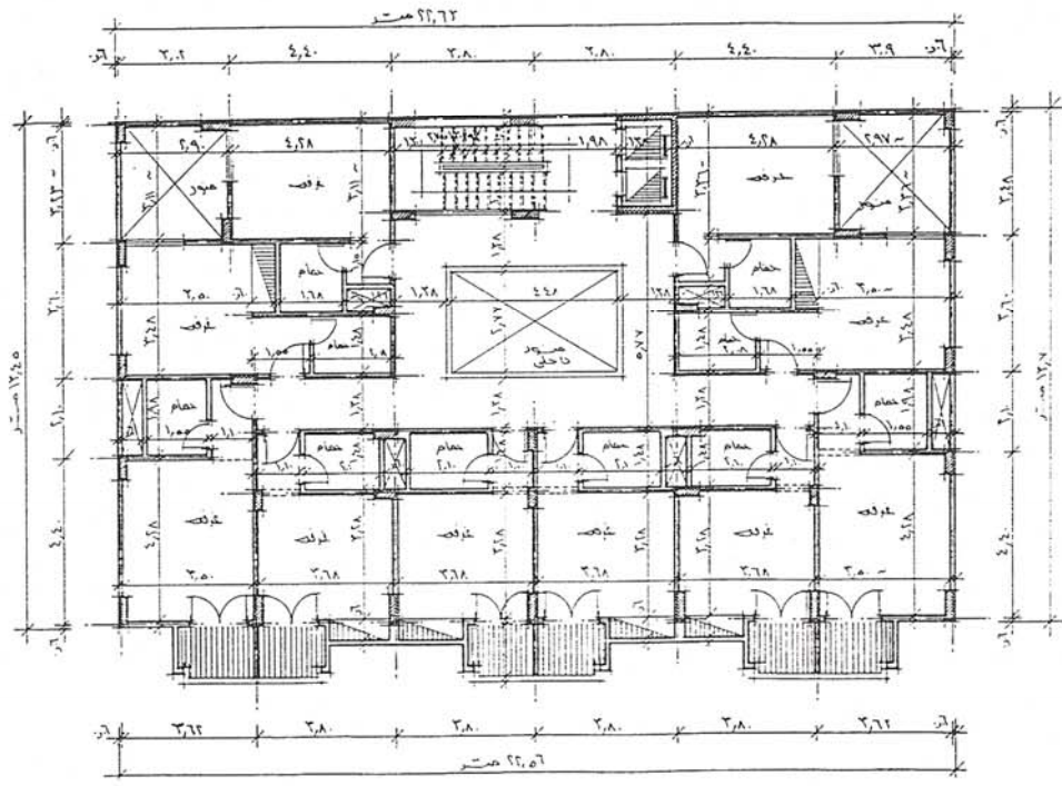
مسقط أفقى للدور المتكرر
