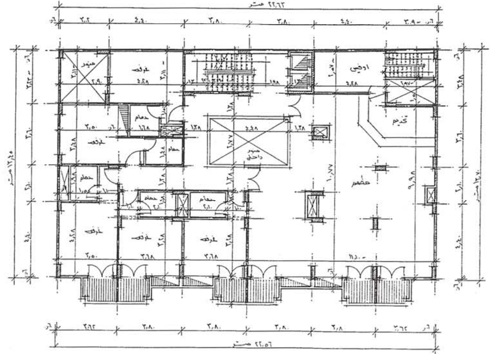
مسقط أفقى للدور الأول العلوى
