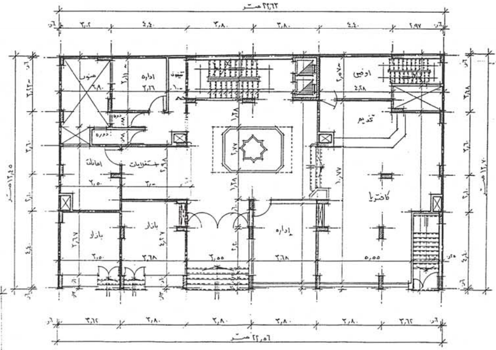
مسقط أفقى للدور الأرضى
