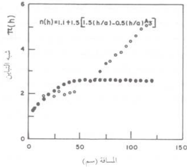
شكل رقم ٤ . علاقة شبه التباين ومسافة التسرب (الدوائر المفتوحة) وعلاقة شبه التباين ومسافة معدلات التسرب المحسوبة باستخدام المعادلة الموضحة على الشكل (الدوائر المغلقة).
